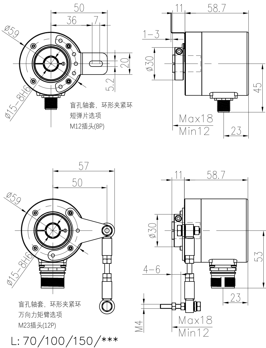
HS25M 外形图
