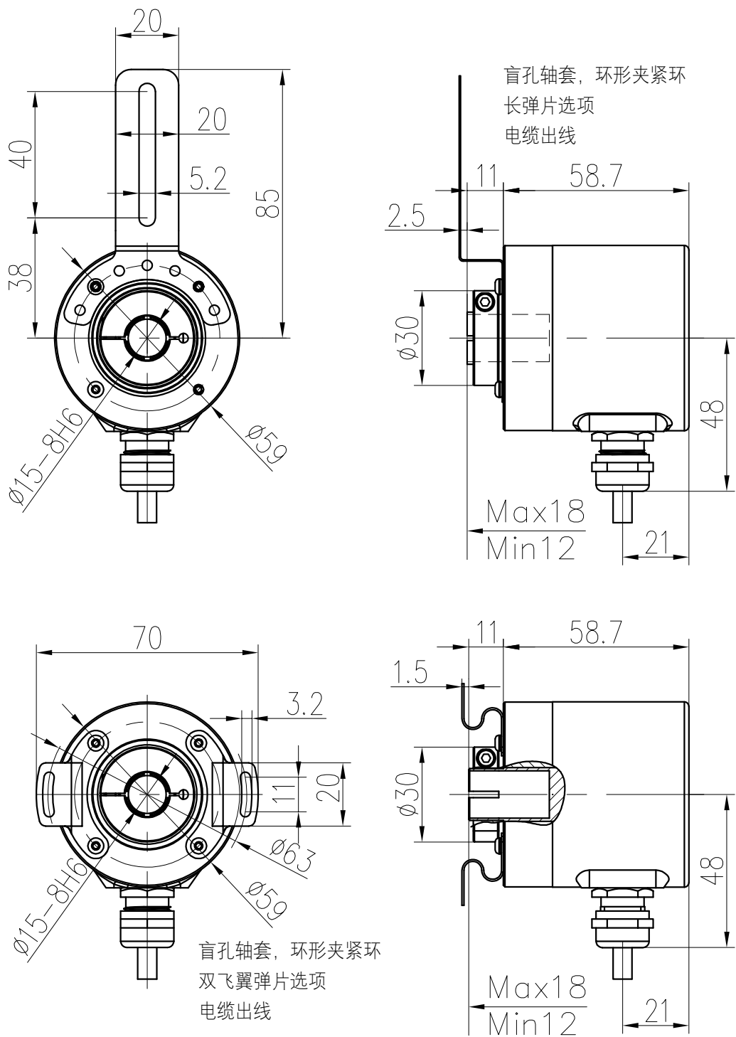
HS25M外形图
