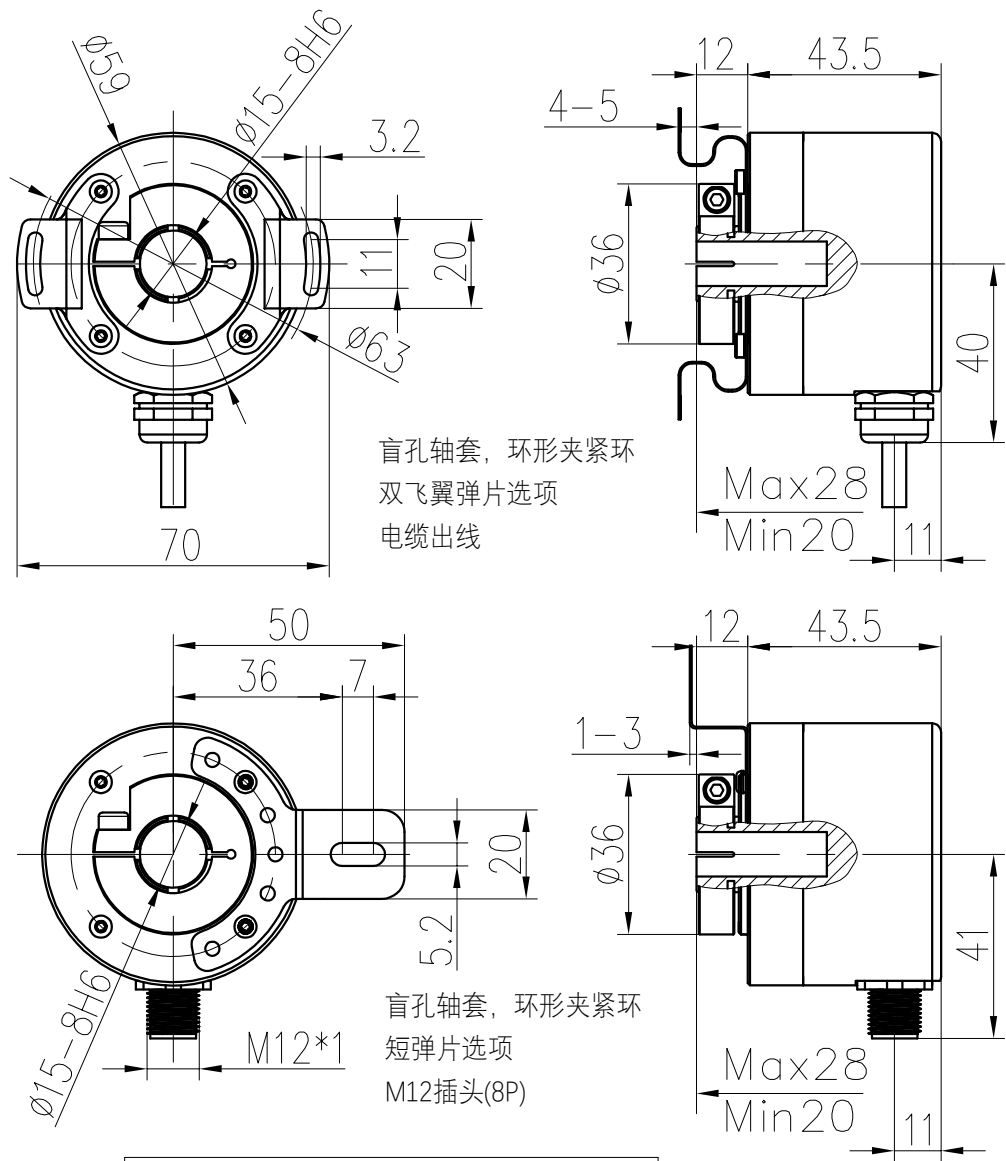
HS25A 外形图
