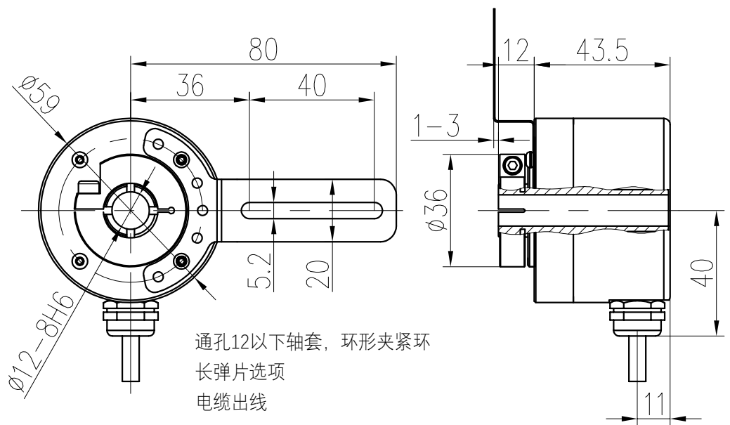
HS25A 外形图
